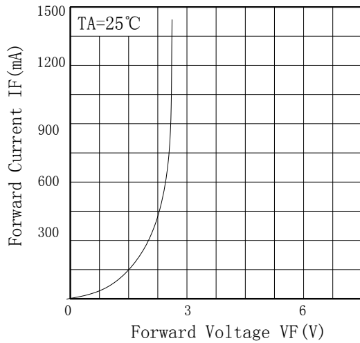
IF - VF
